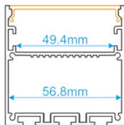
R6060 COD: 7800270
