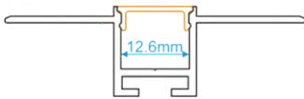
TRL1516 COD: 7800525
